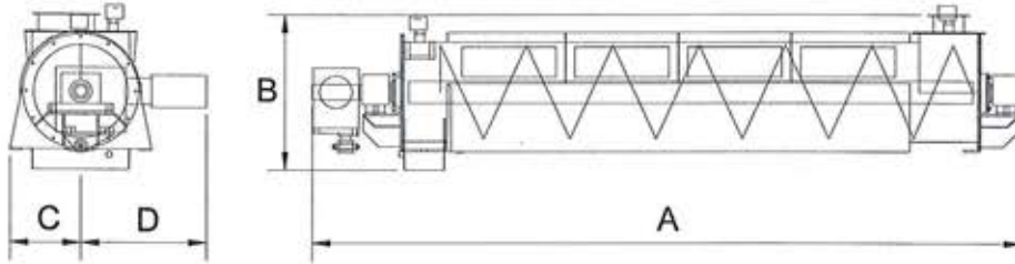
Hygienizáló / Szuperkondicionáló Méretek mm (változtatás joga fenntartva)
