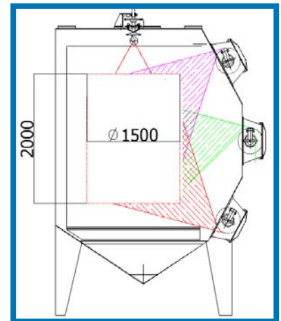
Blast pattern
